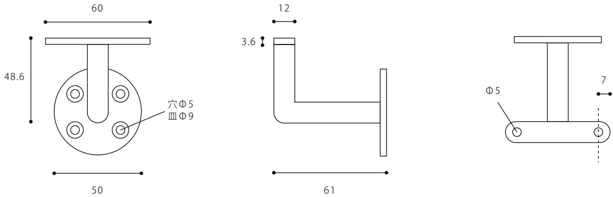
寸法図
